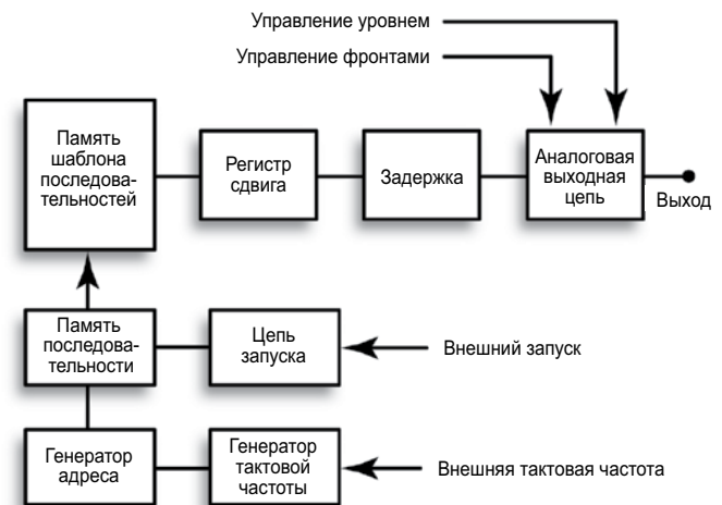
Рис. 41. Упрощенная архитектура PPG или DTG.
