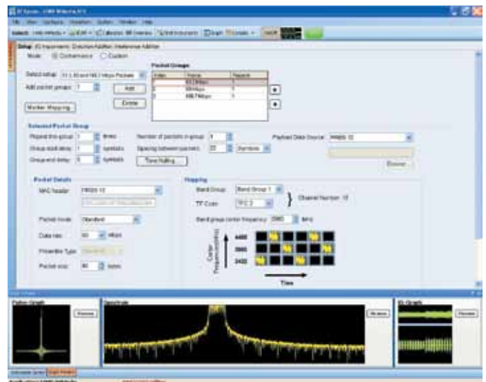
Рис. 40. ПО RFXpress легко создает сложные сигналы со сверхширокой полосой.
