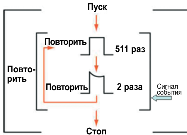
Рис. 32. Объем памяти сигнала AWG можно расширить за счет циклов и повторений.
