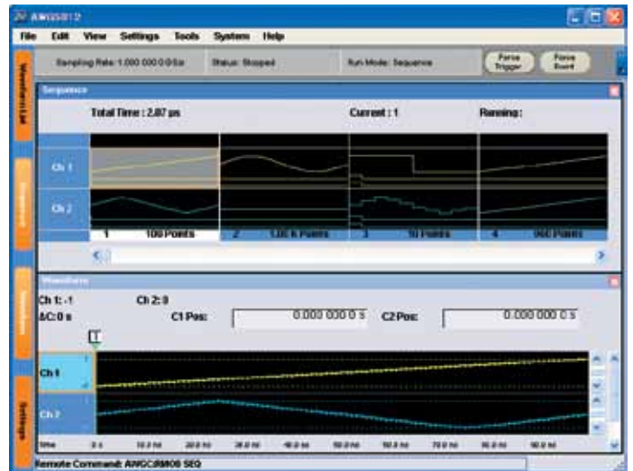
Рис. 33. Для гибкого создания сигналов используется сочетание графического редактора с редактором последовательностей.
