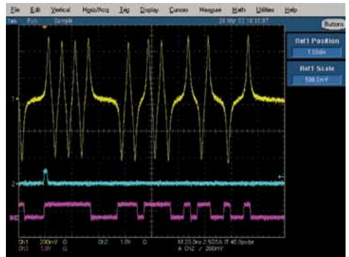
Рис. 29. Выходы маркеров.
