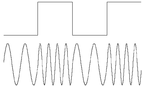
Рис. 13. Частотная манипуляция (ЧМн)
